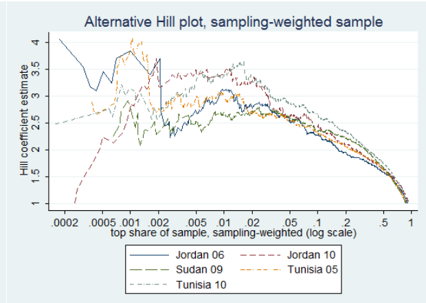
(d) Alternative Hill plots: Jordan, Sudan and Tunisia
