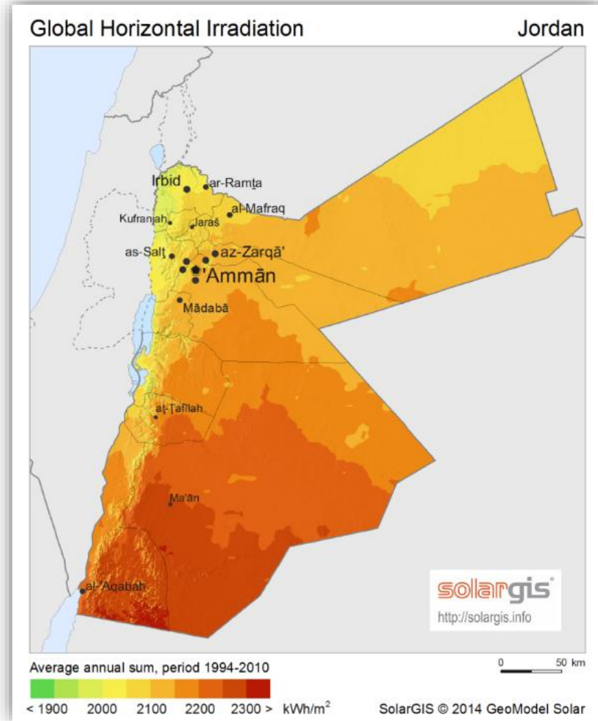
الشكل (14): الإشعاع الشمسي في الأردن
