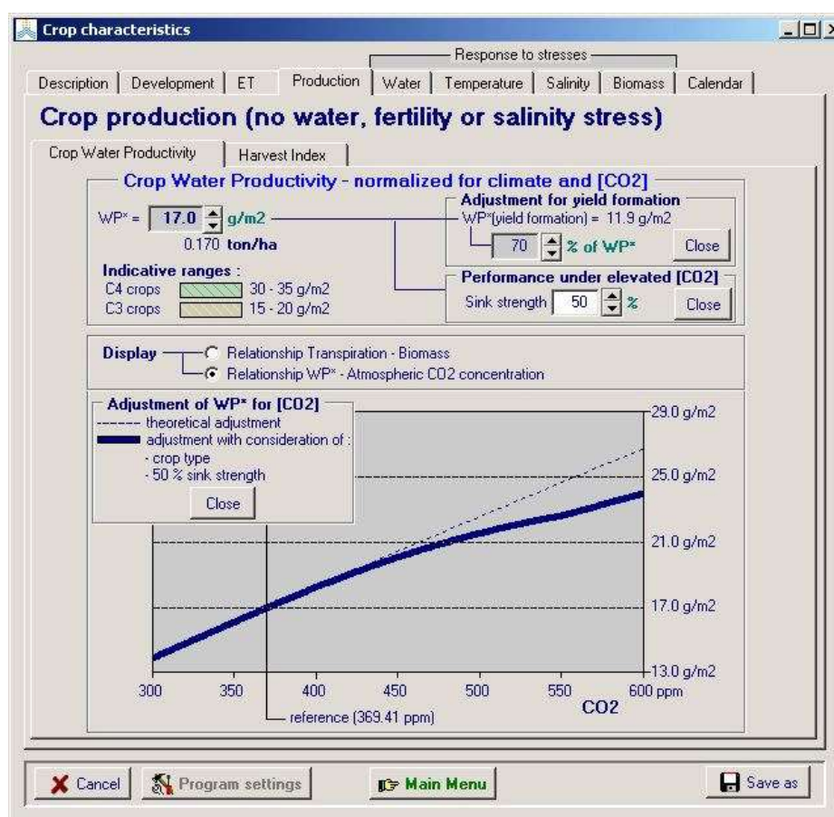
الشكل 10.2h: إنتاجية المياه المعدلة للمحصول من أجل تركيز غاز CO2 في الغلاف الجوي من خلال النظر في نوع المحصول crop type وقوة امتصاص غاز ثاني أوكسيد الكربون أو ما يدعى قوة امتصاص المحصول crop sink strength.
