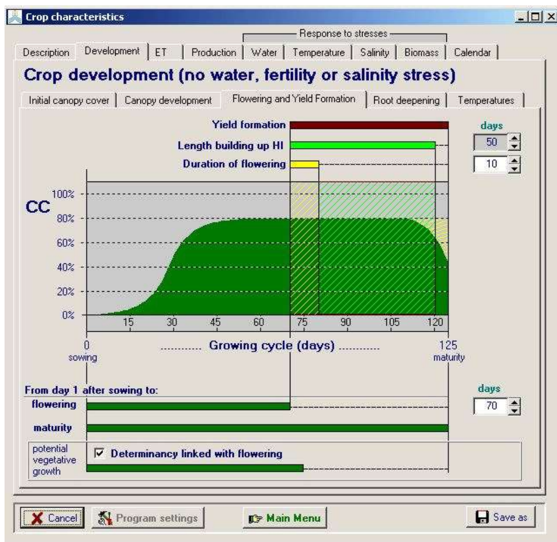
الشكل 5f10.2: مواصفات الإزهار والوقت المطلوب لبناء مؤشر الحصاد لمحاصيل منتجة للثمار أو الحبوب في قائمة خصائص المحصول من أجل محصول ما وذلك عندما يكون التحديد determinacy مرتبطاً مع الإزهار.
