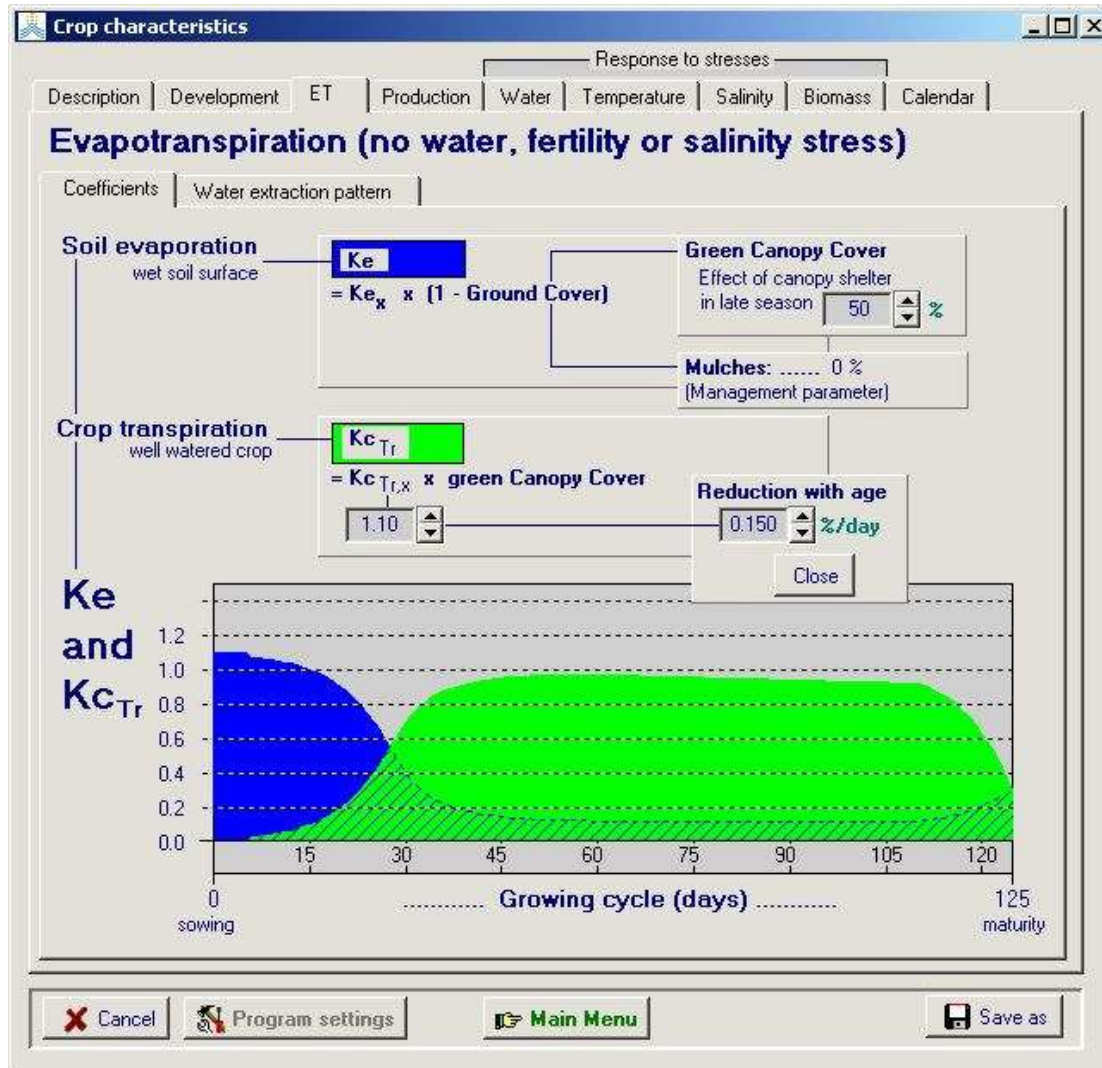
الشكل 1g10.2: يوضح استجابة معامل تبخر التربة ( K_e ) ومعامل نتح المحصول ( K_{CTr} ) لنمو وتراجع الغطاء النباتي canopy خلال دورة النمو وذلك من أجل شروط غير مقيدة non limiting conditions
