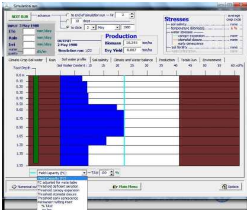
شكل 21.2d: اختيار محتوى مائي محدد للإظهار في واجهة مقطع ماء التربة 'Soil water profile' في قائمة تشغيل المحاكاة Simulation run menu.
