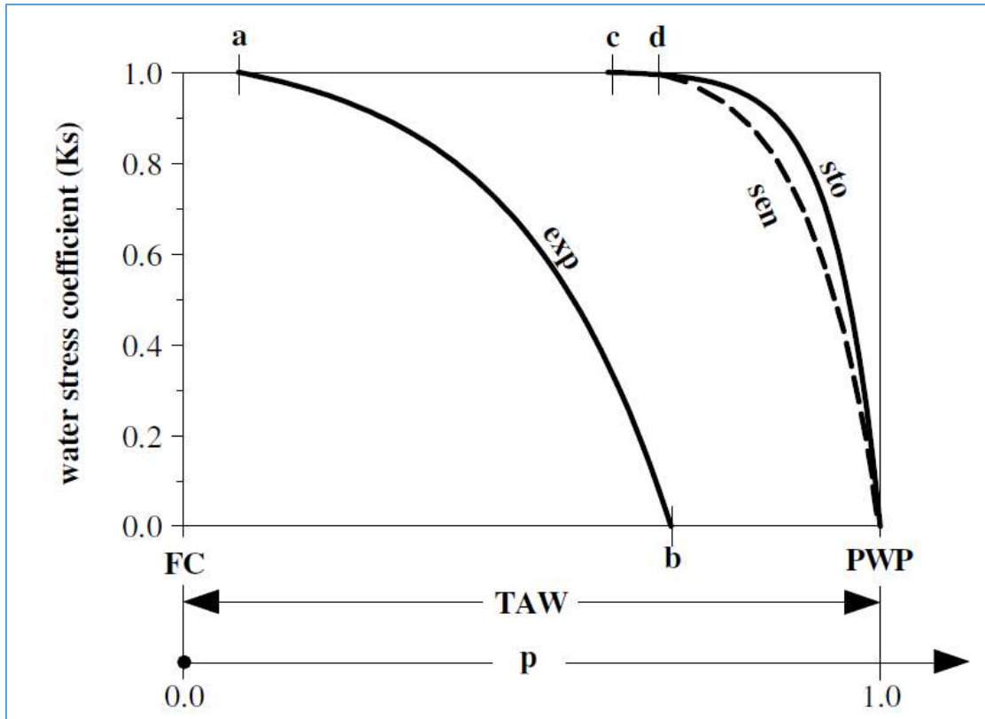
الشكل 10.2: أمثلة على تباينات (تغيرات) معامل الإجهاد المائي Water stress coefficient لتوسع الأوراق stomatal conductance (sto) شيخوخة الغطاء النباتي leaf expansion (exp) وتوصيل المسامات canopy senescence (sen) لاستهلاكات مختلفة لمياه التربة في منطقة الجذور.
