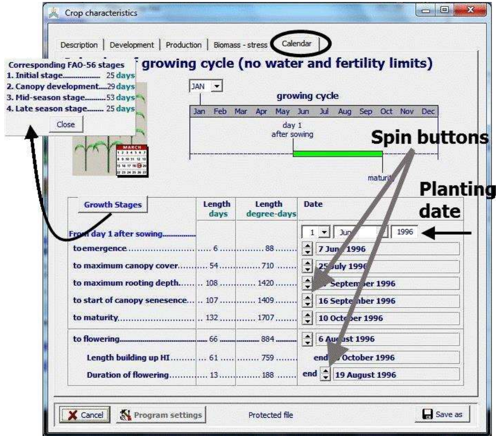
الشكل 10.2.q: الجدول الزمني (تقويم المحصول) لتدقيق وتعديل تقويم النمو، مع الإشارة إلى مراحل النمو لمنظمة الأغذية والزراعة FAO-56.
