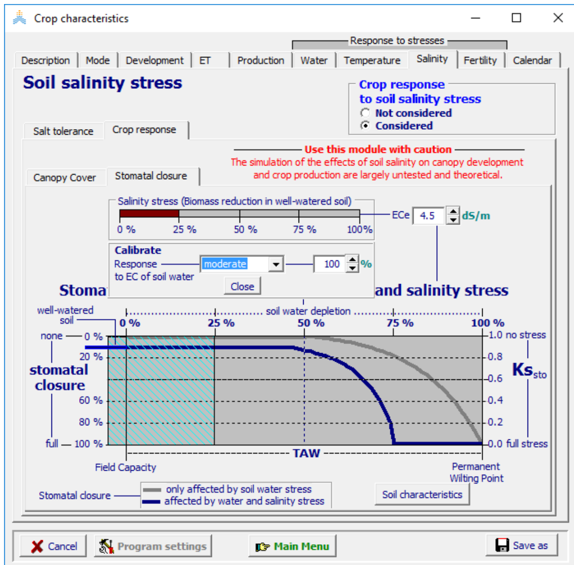
شكل 10.2p5: معايرة تأثير تركيز الأملاح في منطقة جذور مستنفذة على إغلاق المسامات باختيار فئة الاستجابة للنافلية الكهربائية لمياه التربة (EC sw ) أو بتحديد نسبة مئوية للاستجابة في واجهة 'Stomatal closure'
