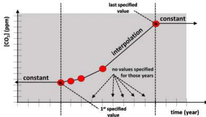
الشكل 2.23c: القواعد التي تنطبق على ملفات CO 2 .
