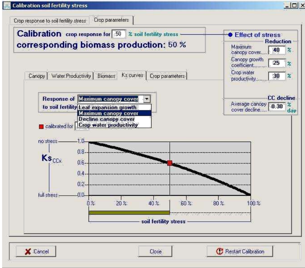
الشكل 10.2m5: منحني Ks من أجل الغطاء النباتي الأعظمي Maximum canopy cover كما هو معروض في واجهة "tab sheet Ks-curves" في قائمة معايرة إجهاد خصوبة التربة Calibration soil fertility stress.
