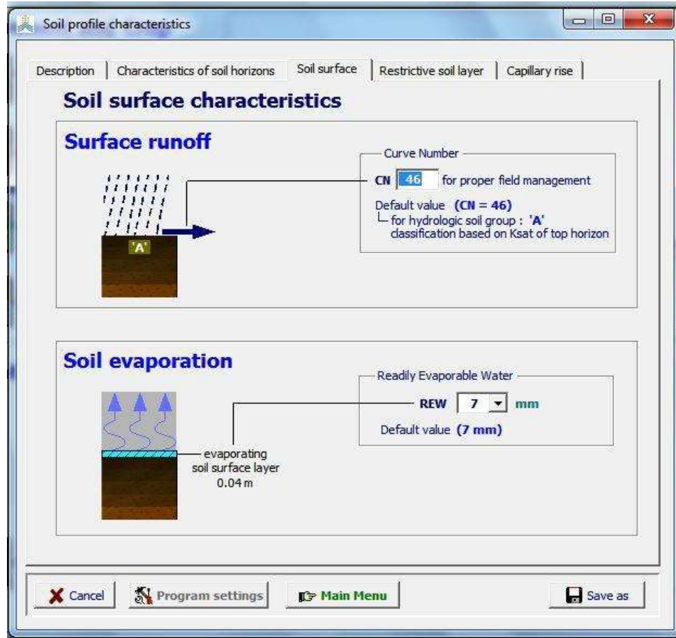
شكل d14.2: خصائص طبقة سطح التربة.
