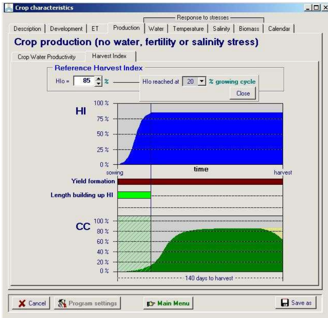
الشكل 5h10.2: مواصفات مؤشر الحصاد والوقت للوصول إلى مؤشر الحصاد المرجعي ( HI_0 ) بالنسبة لمحاصيل الخضر الورقية.
