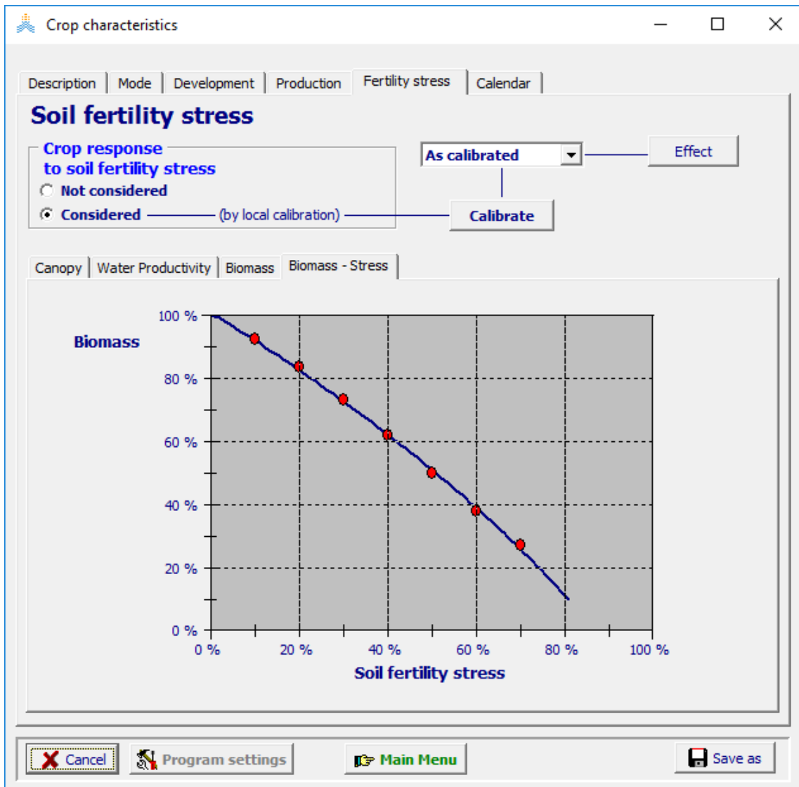
الشكل 6m10.2: عرض للعلاقة بين الكتلة الحيوية وإجهاد خصوبة التربة في واجهة "علاقة الإجهاد بالكتلة الحيوية" Biomass-Stress في قائمة خصائص المحصول.
